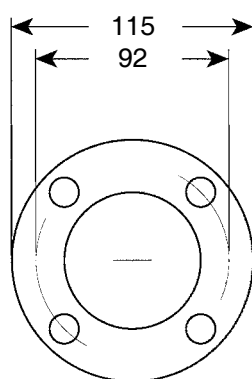
Flangia standard
