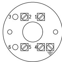
ESECUZIONE SPDT
