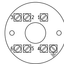
ESECUZIONE DPDT
